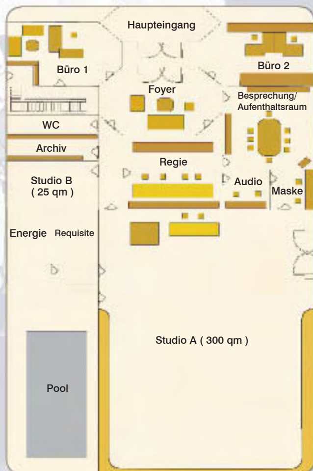
Studiogrundriss
